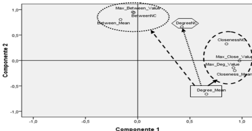
Gráfico de componentes en espacio rotado
